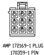
ENCODER CONNECTOR 접속도
