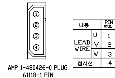
MOTOR CONNECTOR 접속도
